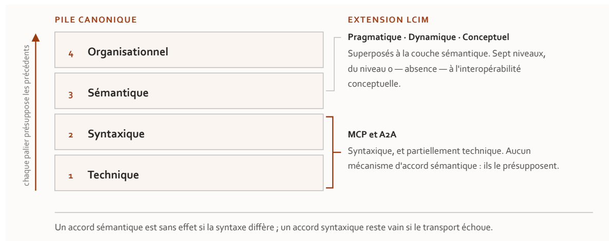
Figure 1.1 — La pile canonique d'interopérabilité, son extension par le LCIM et le palier où opèrent MCP et A2A.
