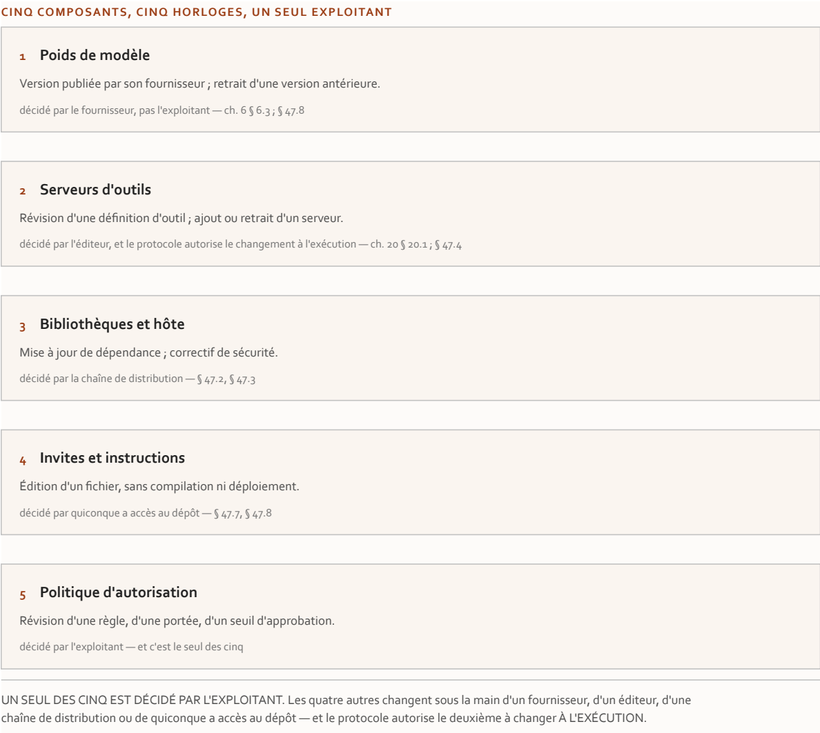
Figure 47.1 — Les cinq composants d'un agent et leurs horloges propres : ce qui les fait changer, et qui en décide.
