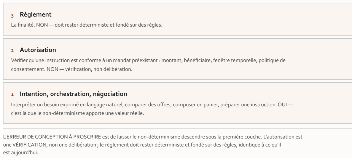
Figure 36.2a — La stratification de la chaîne de paiement, et l'endroit où l'agentique est admise.
