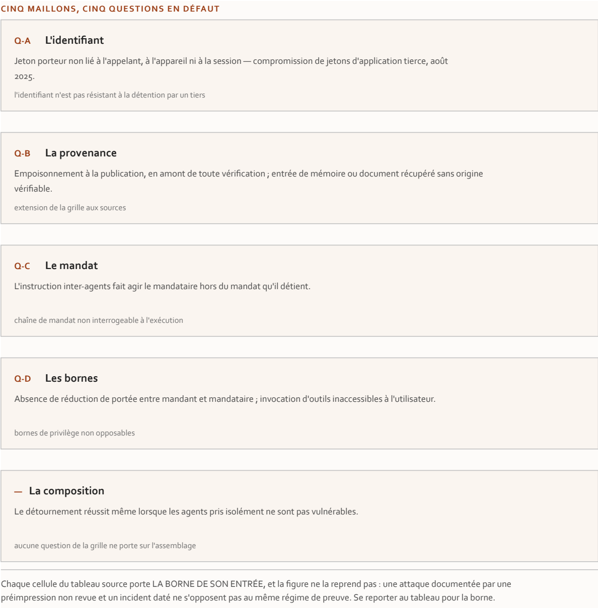
Figure 19.4 — Le tri des attaques par le maillon qui cède, et la question de la grille en défaut.
