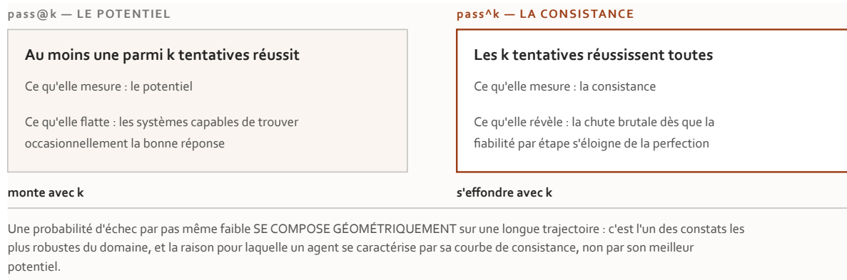
Figure 6.4 — Potentiel contre consistance : deux métriques dont la confusion masque l'effondrement.
