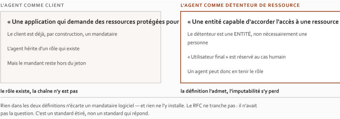
Figure 12.4 — L'agent dans OAuth : client ou détenteur de ressource ? Les deux placements, et ce que chacun engage.
