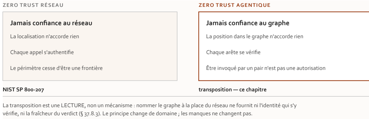
Figure 37.7 — Zero trust transposé : de « jamais confiance au réseau » à « jamais confiance au graphe ».
