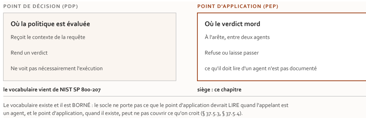
Figure 37.5 — Où se prend la décision d'autorisation, et où elle s'applique.
